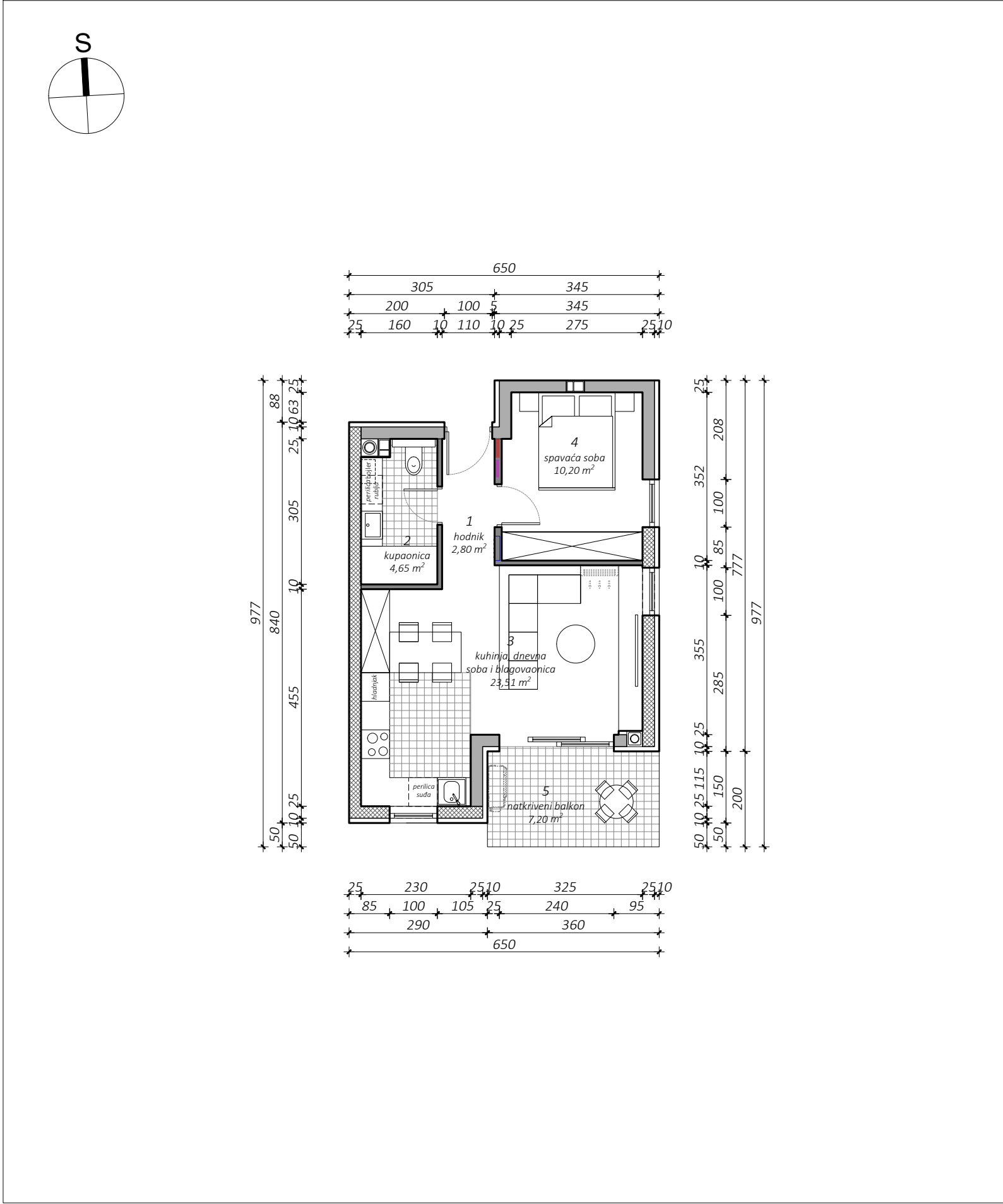
HEMA DILATACIJA - TLOCRT KARAKTERISTIČNE ETAŽE br. prostorija m 2 k k x m 2 POSEBNI DIO 1 hodnik 2,80 1,00 2,80 2 kupaonica 4,65 1,00 4,65 3 kuhinja, dnevna soba i blagovaonica 23,51 1,00 23,51 4 spavaća soba 10,20 1,00 10,20 5 natkriveni balkon 7,20 0,50 3,60 Ukupno posebni dio: 48,36 44,76 SPOREDNI DIO 6 spremište S23 1,75 0,50 0,88 7 GPM 63 12,50 0,60 7,50 Ukupno sporedni dio: 14,25 8,38 Ukupno NP stana 62,61 m 2 Ukupno NKP stana 53,14 m 2 sadržaj: mjerilo: datum: list broj: KATALOG STANOVA STAN A - 23 1:100 rujan 2024. 32
