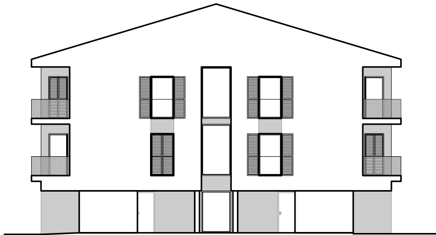
JUGOZAPADNO PROČELJE
