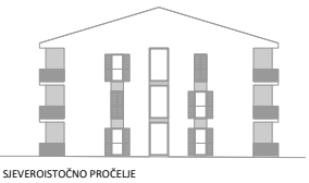
SIJEVEROISTOČNO PROČELJE
