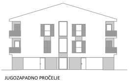
JUGOZAPADNO PROČELJE
