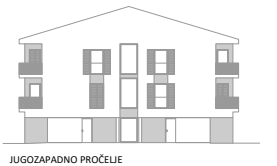
JUGOZAPADNO PROČELJE
