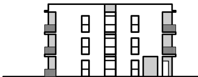
JUGOISTOČNO PROČELJE
