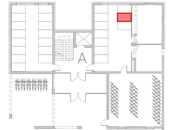
TLOCRT PRIZEMLJA (DILATACIJA A) POLOŽAJ SPREMIŠTA
