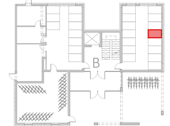
TLOCRT PRIZEMLJA (DILATACIJA B) POLOŽAJ SPREMIŠTA
