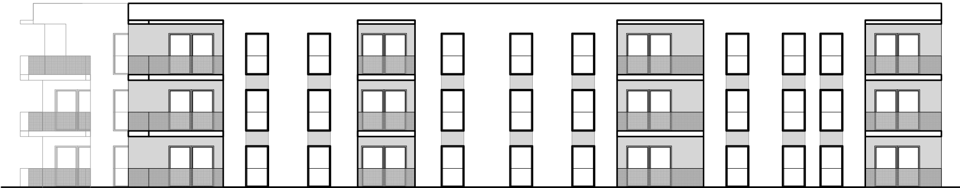
SJEVEROISTOČNO PROČELJE
